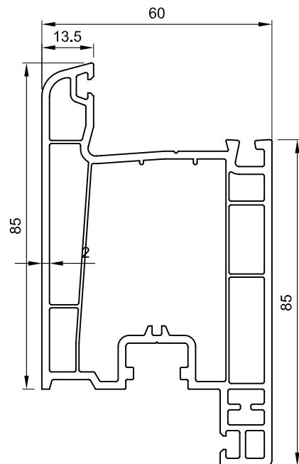
657 Kapı Kanat Profili / Door Sash Profile / بروفایل مصراع الباب 1,340 kg/m
